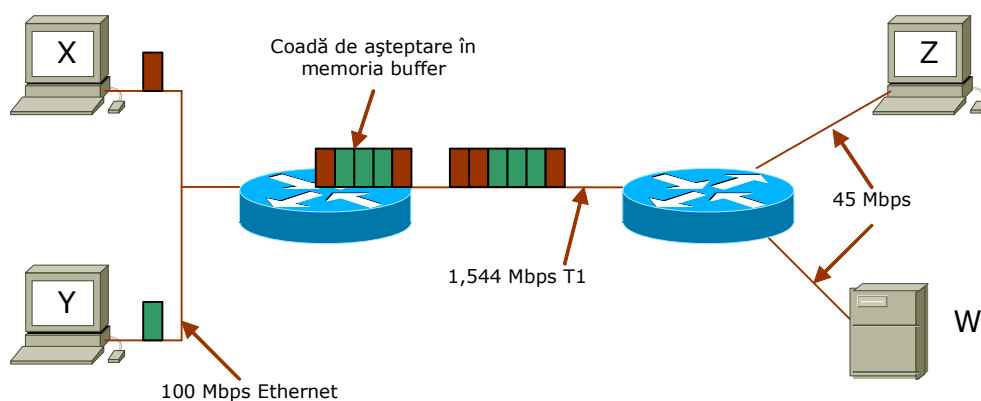
Figura 1.8 Rețea bazată pe comutare de pachete
